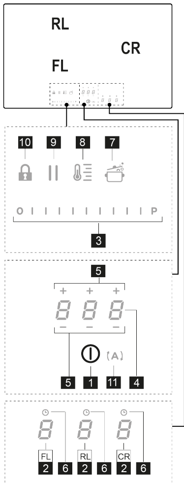
Panel sterowania mod.603
